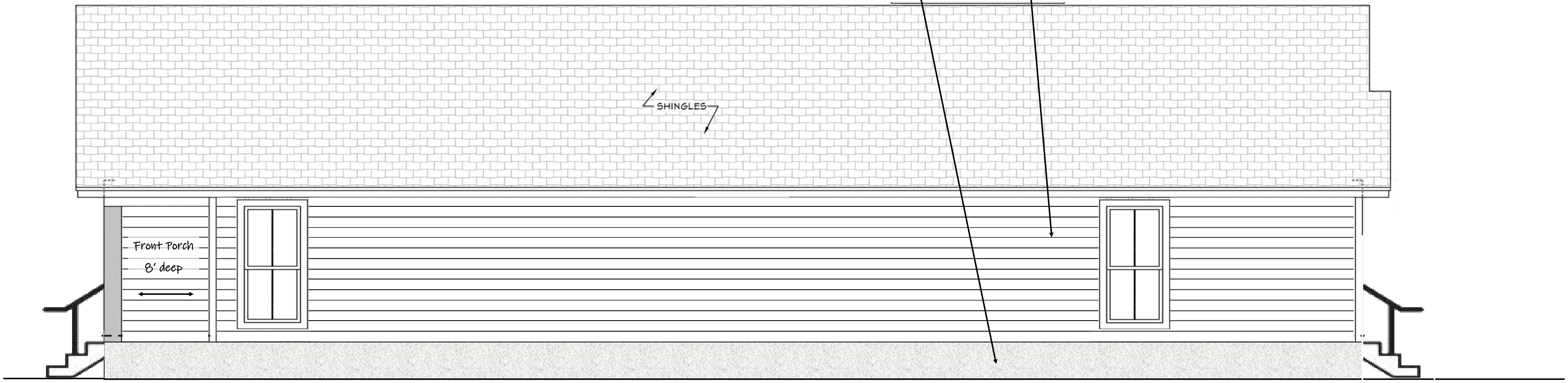
Right Elevation
