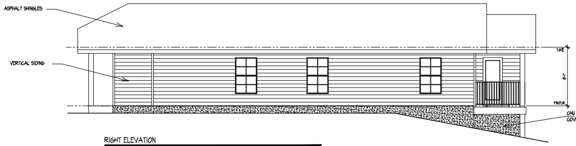
RIGHT ELEVATION
