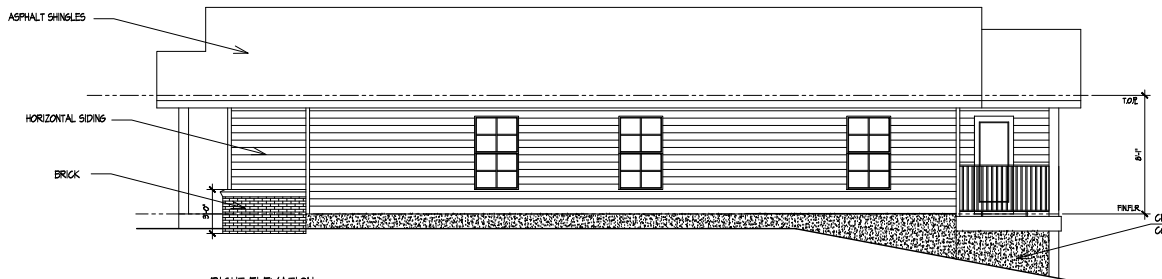
RIGHT ELEVATION
